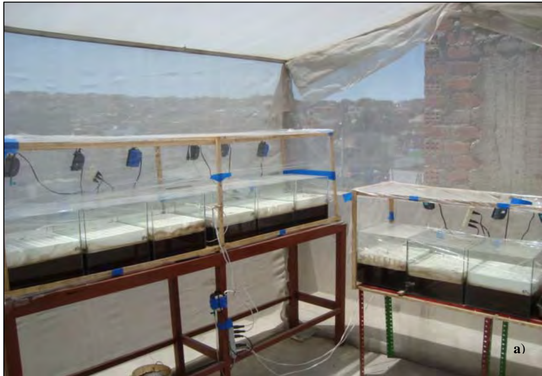
FIGURA 6.1. a) Instalación de experimento final para la bioacumulación de selenio (IV) utilizando Bacopa monnieri L. (Hisopo de agua) bajo condiciones de invernadero
