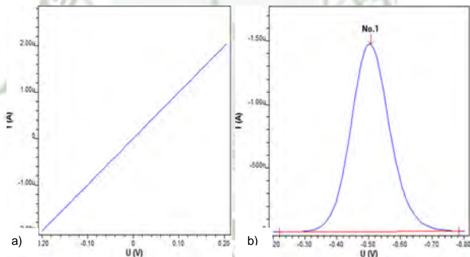
FIGURA 4.1. a) Gráfico lineal expresado en función de la intensidad de corriente (A) y la rampa de voltaje (V), b) Voltamperograma expresado en función de la intensidad de corriente (A) y la rampa de voltaje (V).
