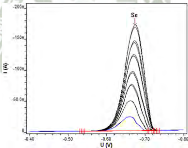
FIGURA 2.2. Voltamperograma con un incremento de picos simétricos que están en función de la intensidad de corriente (A) y la rampa de voltaje (V).
