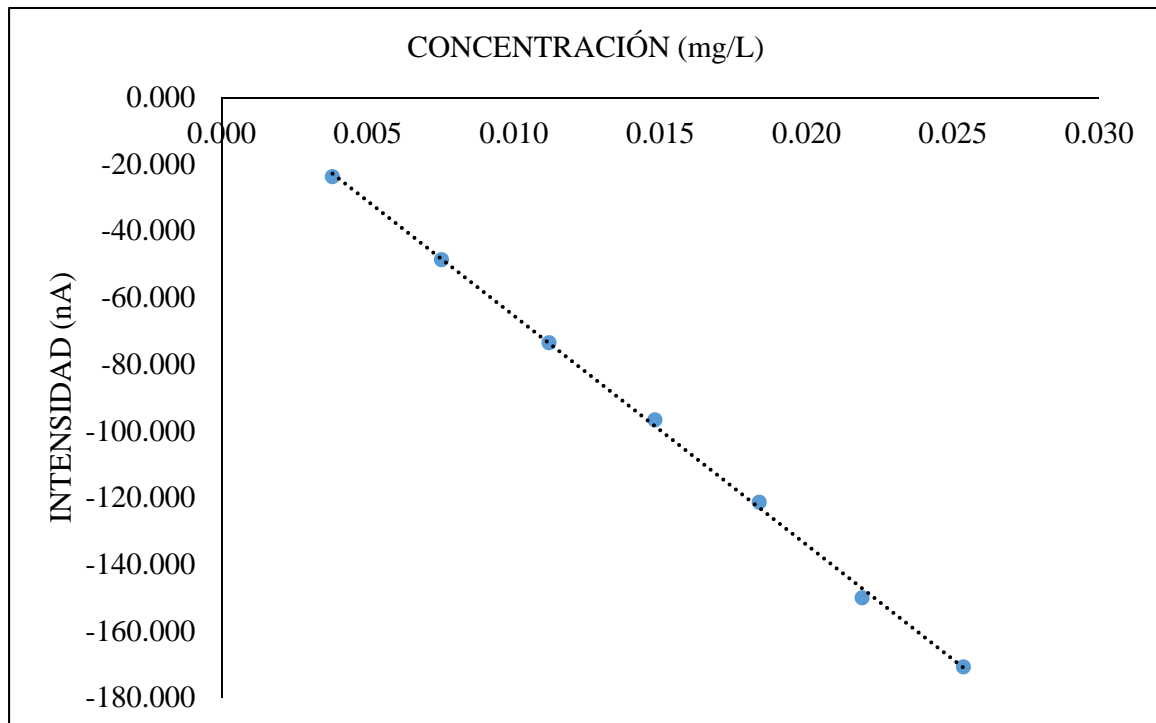
FIGURA 4.3. Representación gráfica de la linealidad del método para la determinación de selenio (IV).
