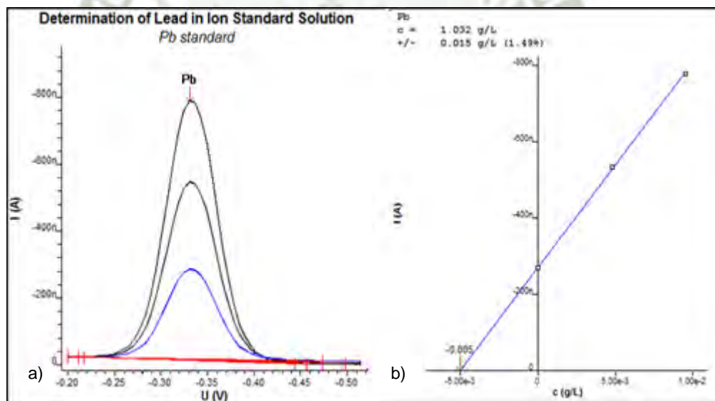
FIGURA 4.2. a) Voltamperograma expresado en función de la intensidad de corriente (A) y la rampa de voltaje (V); b) Gráfico lineal expresado en función de la intensidad de corriente (A) y la rampa de voltaje (V).
